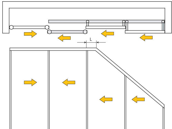
4 deurskast met 2 schuine deuren
